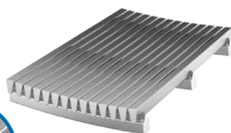
Spaltsieb Gewickelte Profilstäbe mit Stützstäben, Widerstandsgeschweißte Konstruktion
