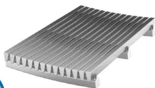
Spaltsieb Gewickelte Profilstäbe mit Stützstäben, Widerstandsgeschweißte Konstruktion
