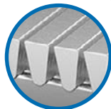
Spaltsieb Gewickelte Profilstäbe mit Stützstäben, Widerstandsgeschweißte Konstruktion
